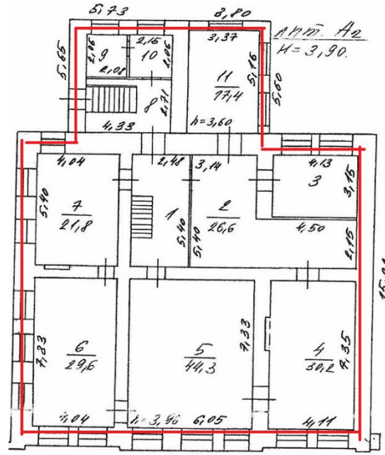
План 2 этажа*
