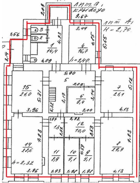
План 1 этажа*
